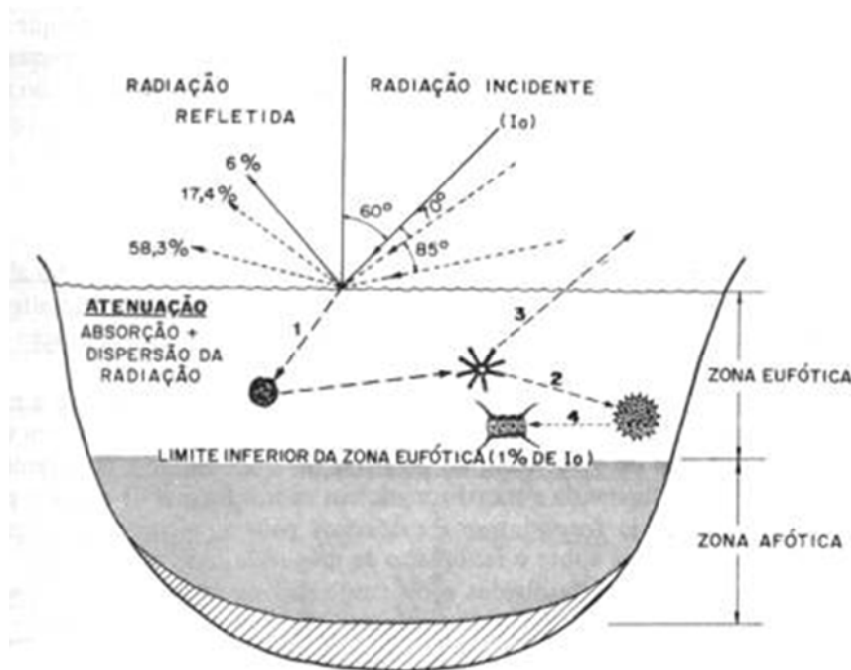
Figura 29 – Diagrama mostrando o comportamento da radiação solar em um ambiente aquático.
