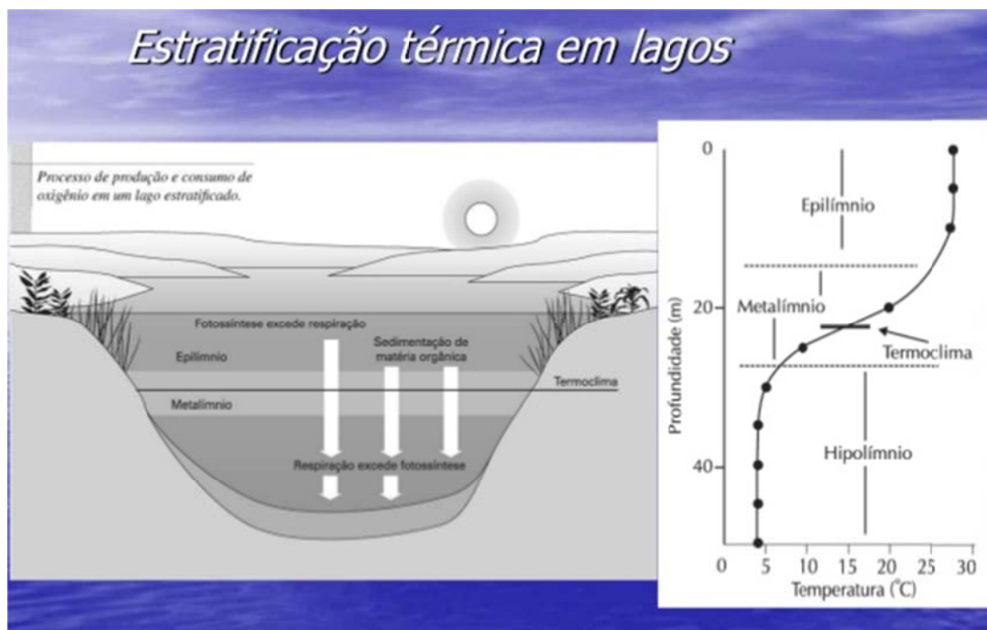
Figura 36 – Esquema mostrando a Estratificação Térmica em Lagos
