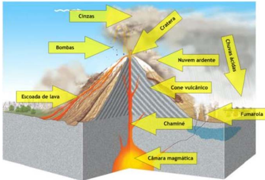
Figura 50 – Alguns aspectos da atividade vulcânica.
