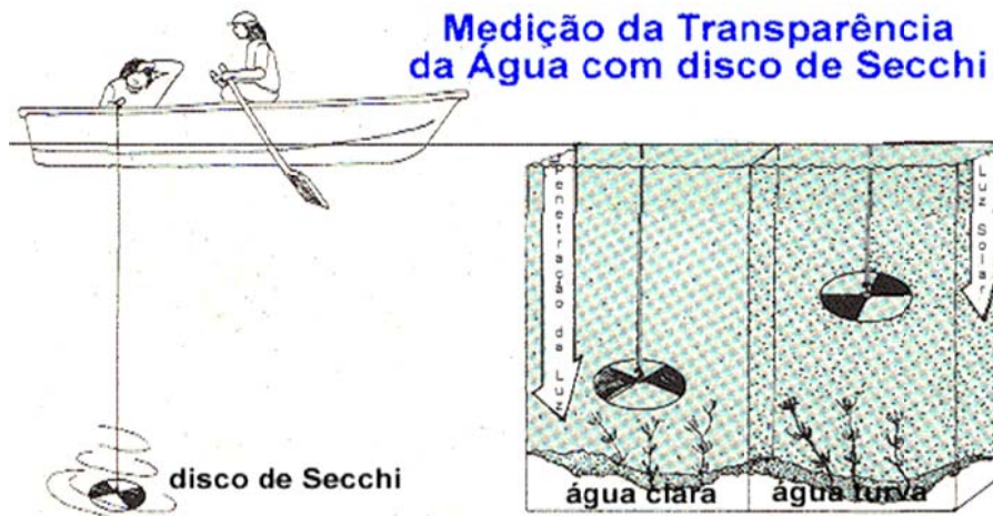
Figura 35 B – Esquema com a Medição da Transparência da Água com disco de Secchi.
