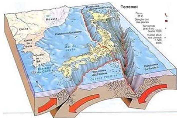
Figura 1 – Esquema da gênese tectônica
