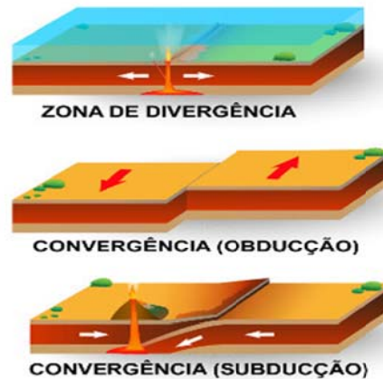
Figura 2 – Tipos de zonas de tensão tectônica
