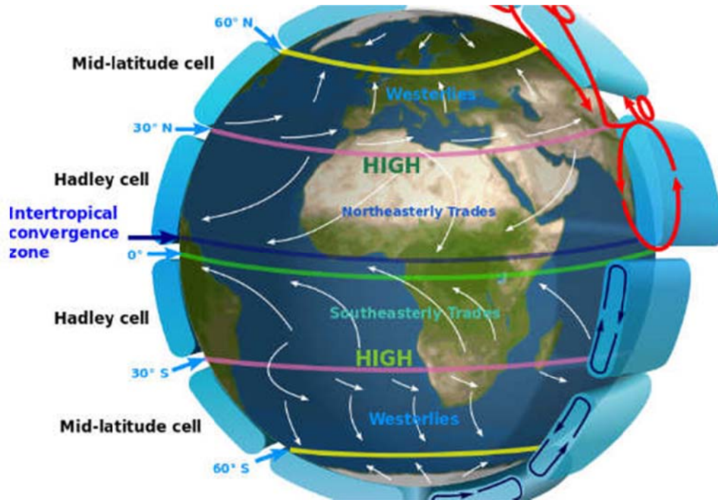
Figura 48 - Exemplo simplificado da dinâmica atmosférica do Planeta.
