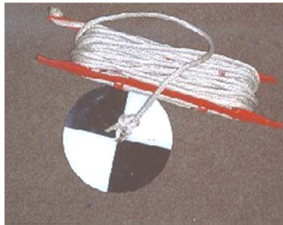
Figura 35 A – Disco de Secchi atado com corda graduada.
