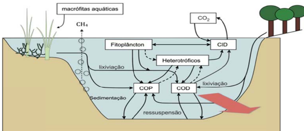
Figura 38 – Exemplo de algumas interações relativas ao elemento carbono
