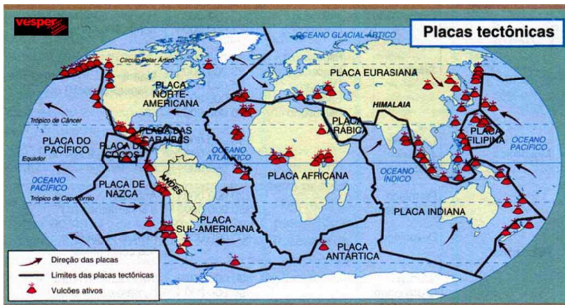
Figura 47 – Desenho esquemático das principais placas tectônicas do Planeta.
